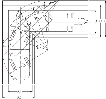
●4輪ステアリングで右折する場合
